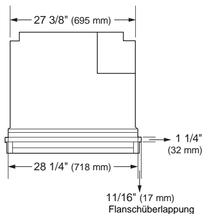
Typischer Einbau-Backofen (Einzelgerät)
